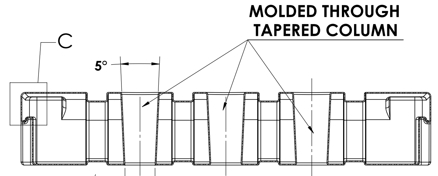
SECTION A-A SCALE 1 : 14
